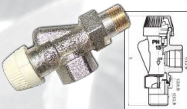
Клапан радиаторный регулирующий осевой
