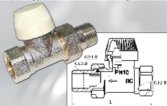
Клапан радиаторный регулирующий прямой
