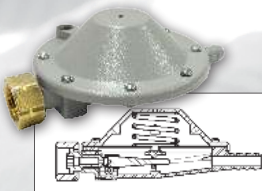
РДСГ 1-1,2 "Лягушка"
